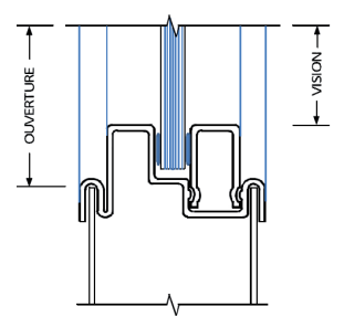
KIT DE MOULURE "SI"
