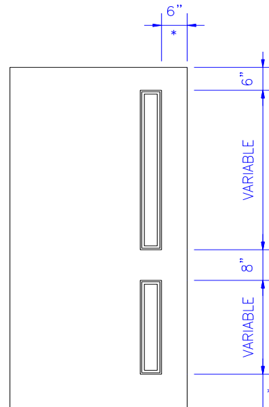
TYPE "DNL"
