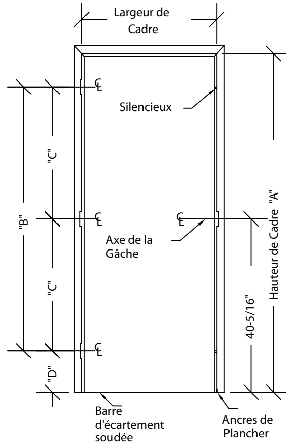
ÉLÉVATION
