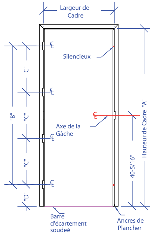
ÉLÉVATION
