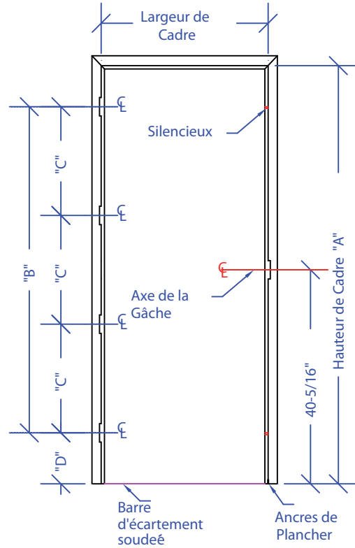
ÉLÉVATION
